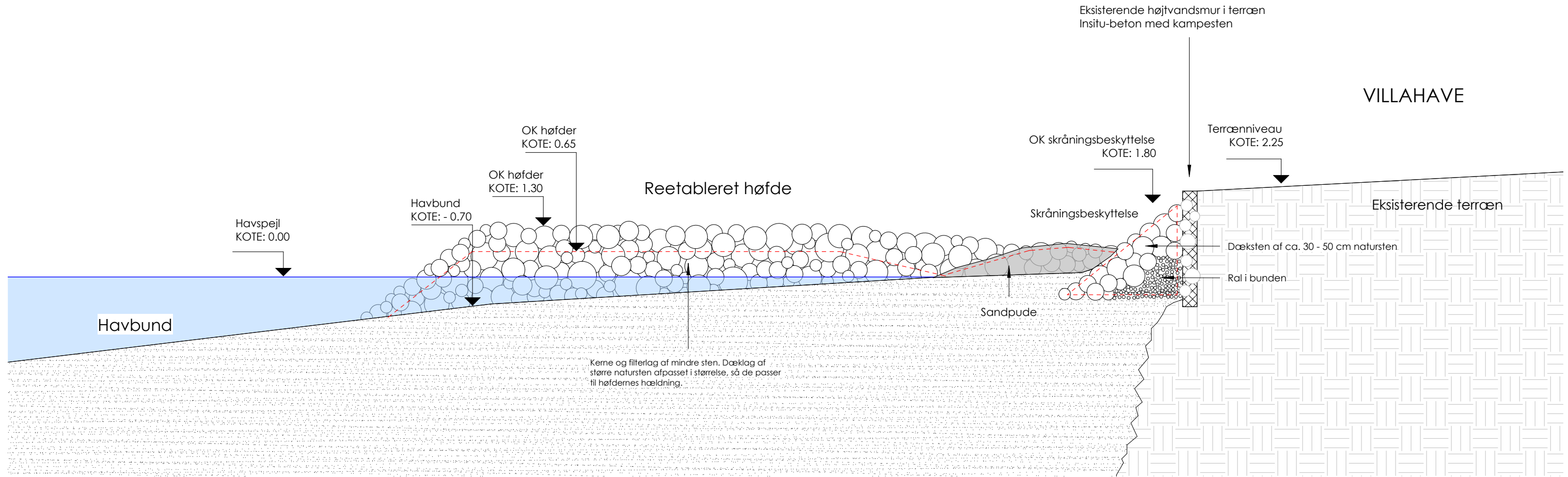
SNIT A-A 1 : 100
